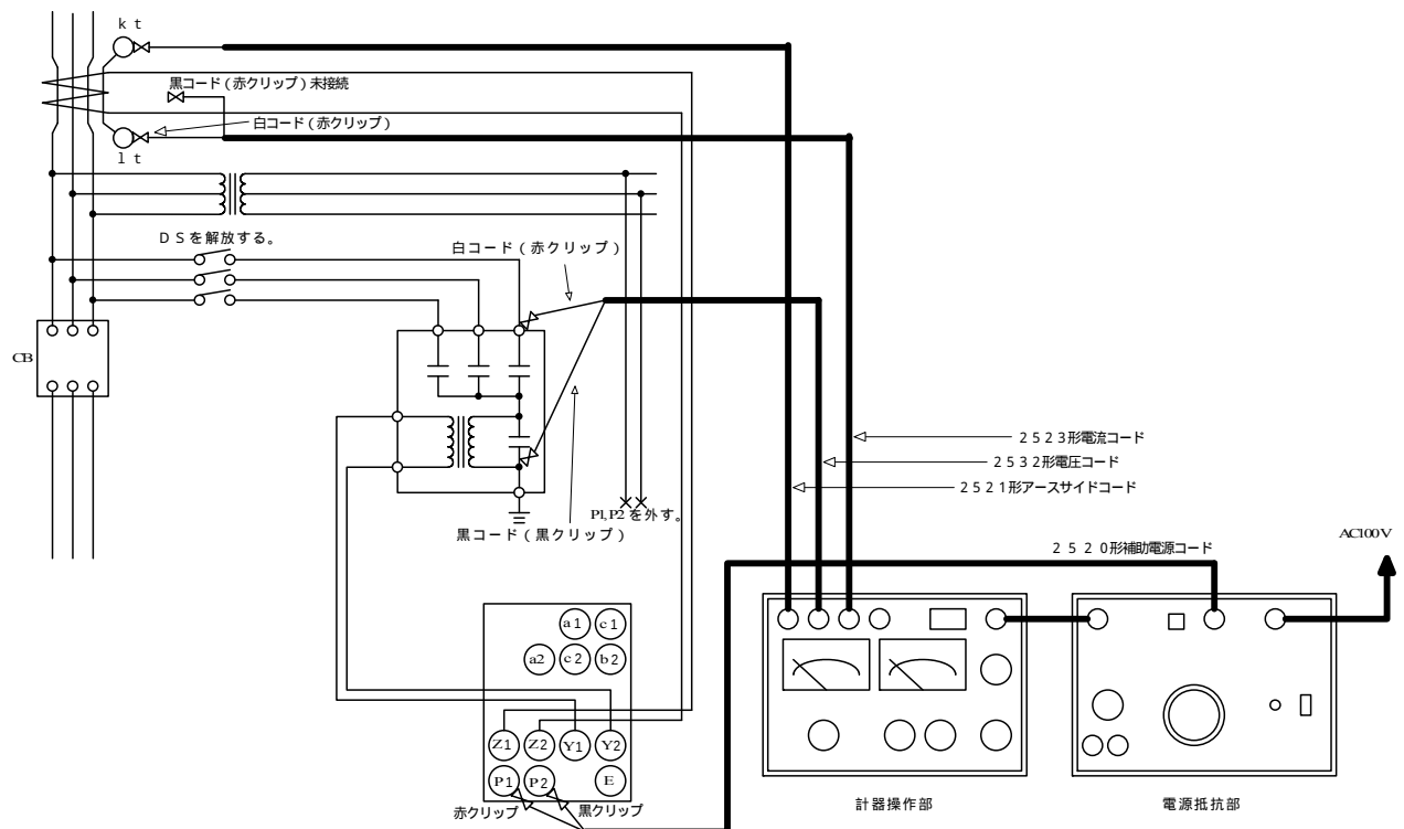
結線図
