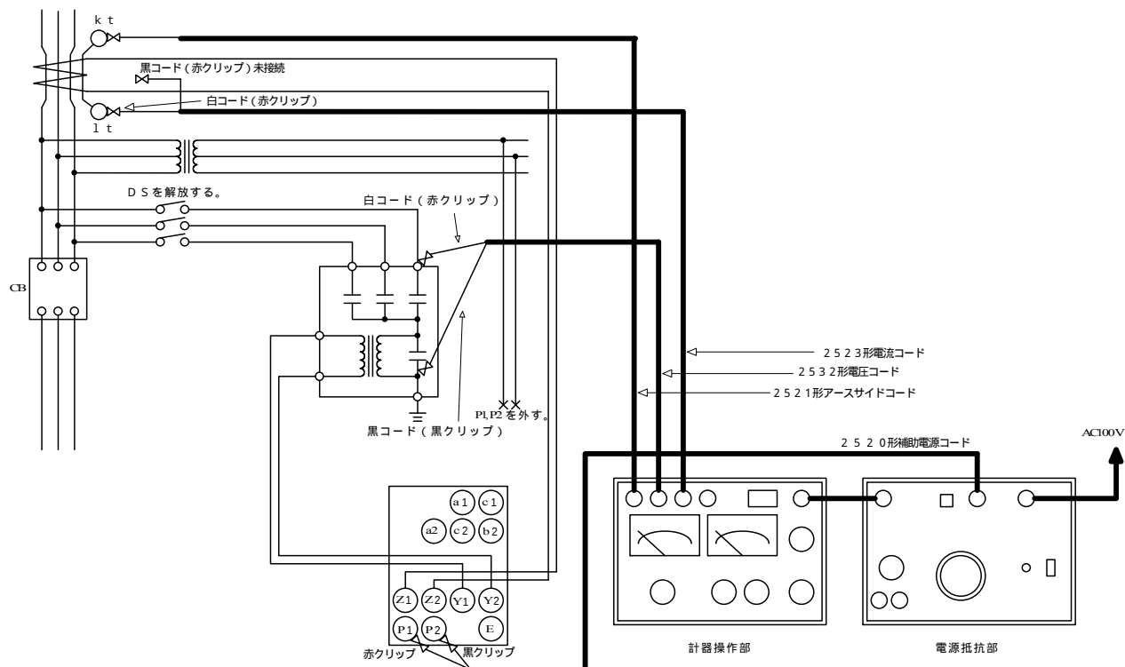
結線図
