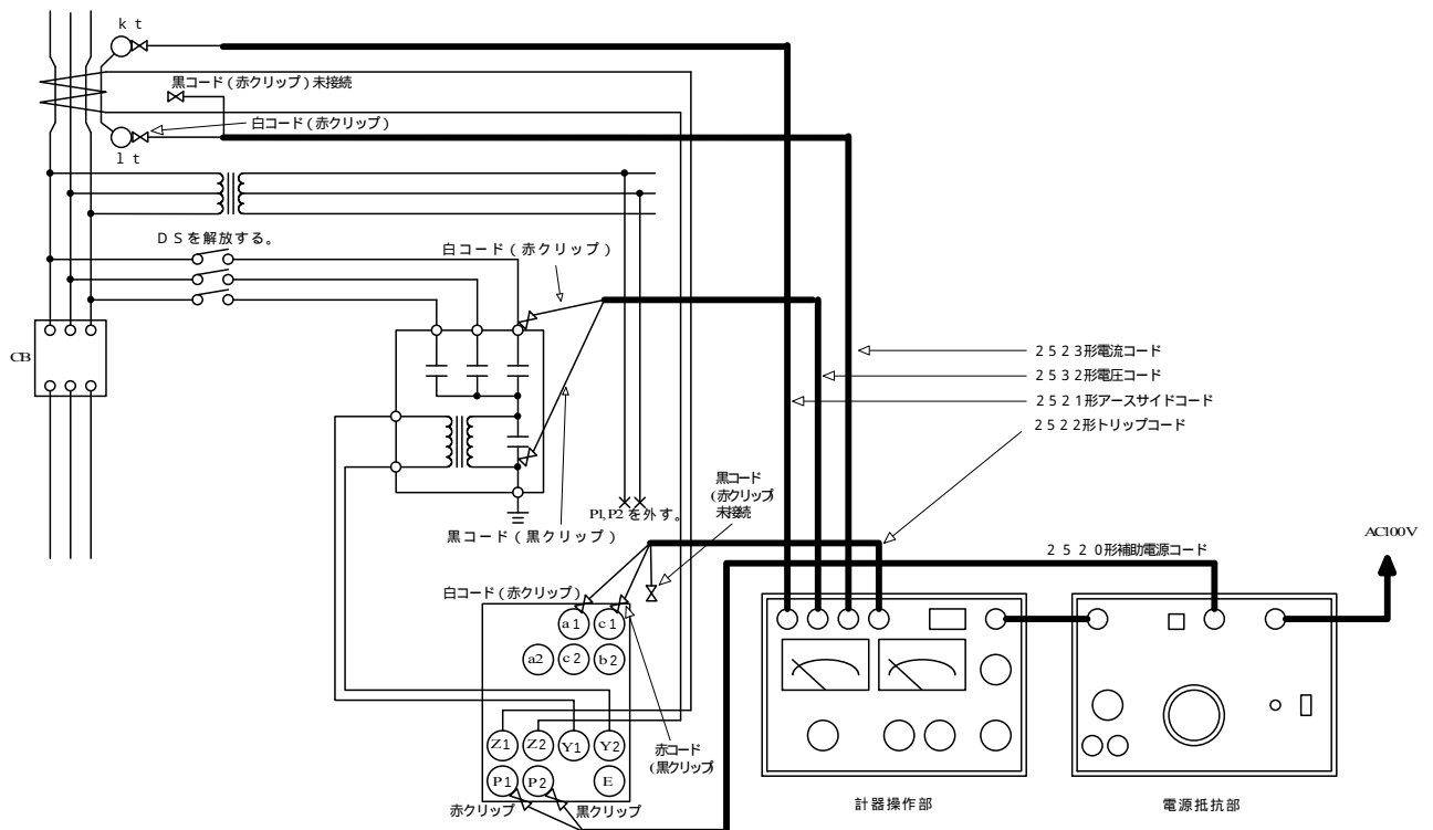
結線図
