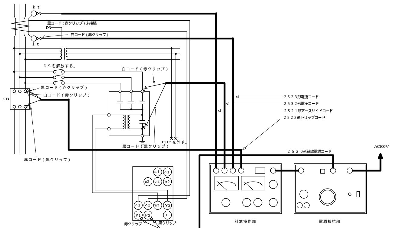
結線図
